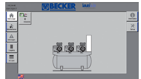
Vakuumsystem med oliesmurte lamel-vakuumpumper og tank
