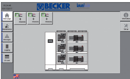
VARI AIR central System met zijkanaalventilatoren en schottenvacuümpompen
