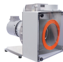
RV 2.1944/10 incl. filtro de succión
