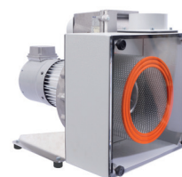
RV 2.1944/10 흡기 필터 포함
